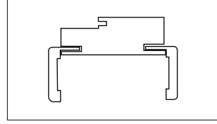
Düz Kasa Ölçüleri Door Frame Sizes
